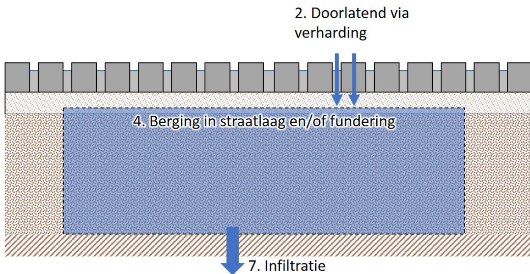
Figuur 2-4: Schematisatie Aquaflow regular als infiltrerend system
